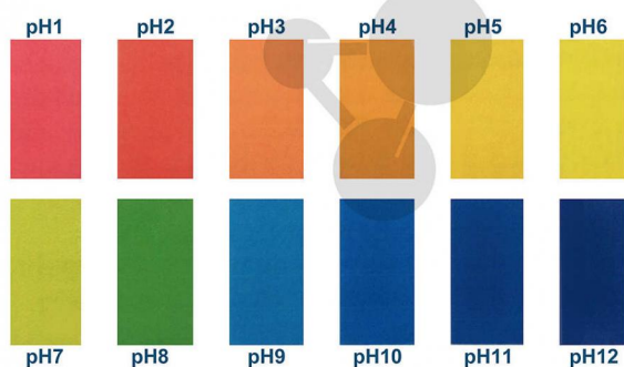
pH-Farbskala zum Universalindikator
